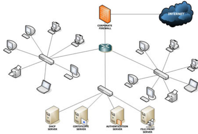
ნახაზი 14. ლოკალური ქსელები – Local Area Networks (LAN)
